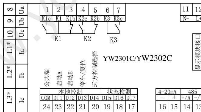
YW2301C/YW2302C 接线端子示意图
