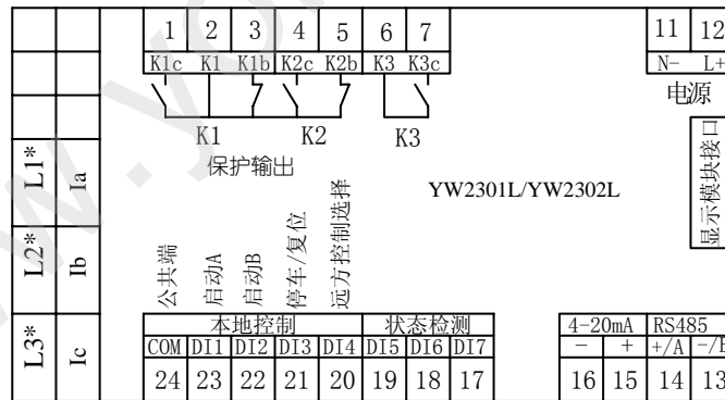
YV2301L/YV2302L 接线端子示意图
