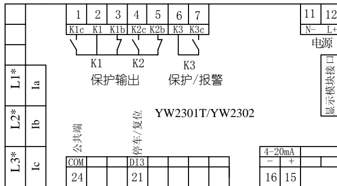
YV2301T/YV2302T 接线端子示意图
